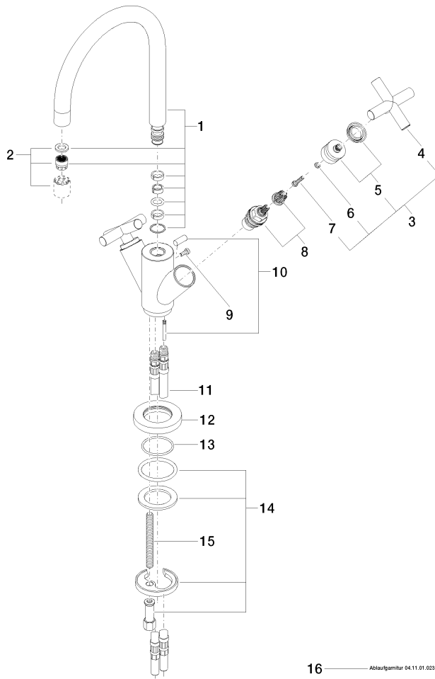
16 ——— Ablaufgarnitur 04.11.01.022.00-ff
